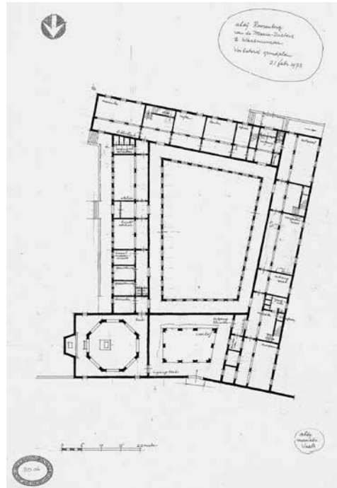
Plan voor Roosenberg (1973), archief Van der Laan-stichting.
