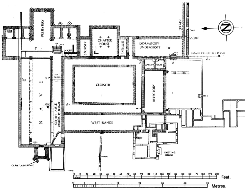
Plattegrond van de absite Boxley (1952) en plan van het klooster (1973).
